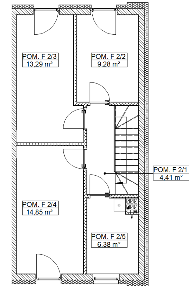
Rzut piętra:
