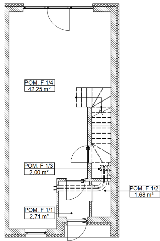
Rzut parteru:
