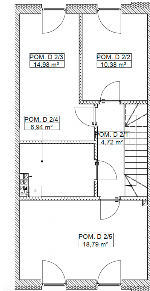
Rzut piętra:
