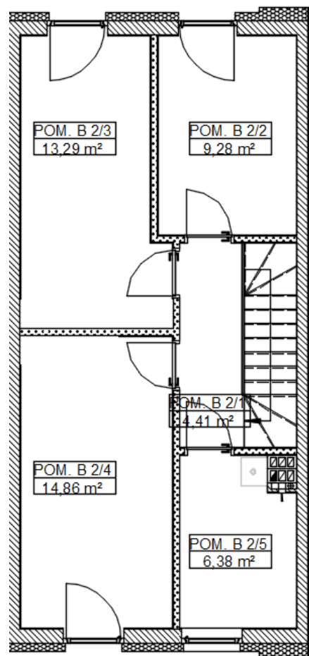
Rzut piętra:
